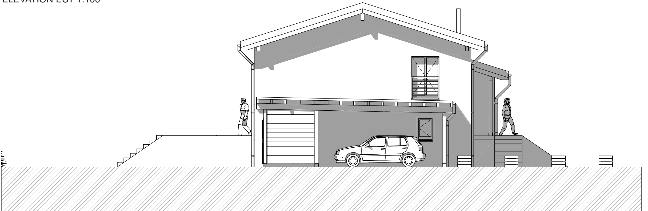
ELEVATION EST 1:100
