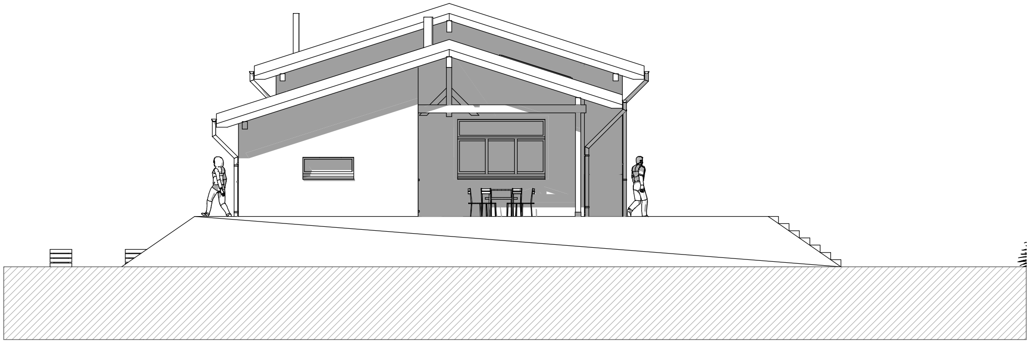
ELEVATION OUEST 1:100
