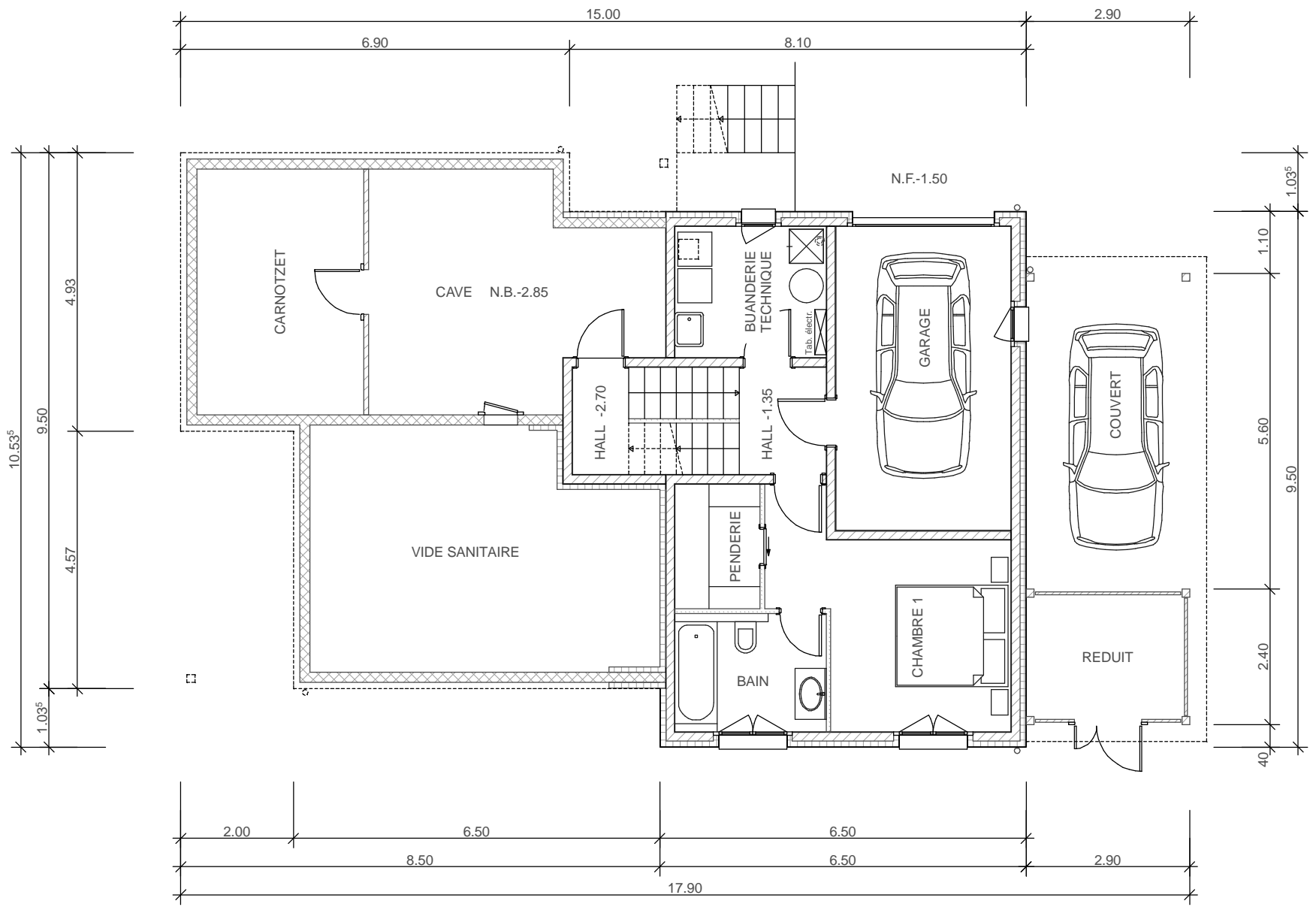
NIVEAUX DU SOUS-SOL ET REZ INFÉRIEUR 1:100
