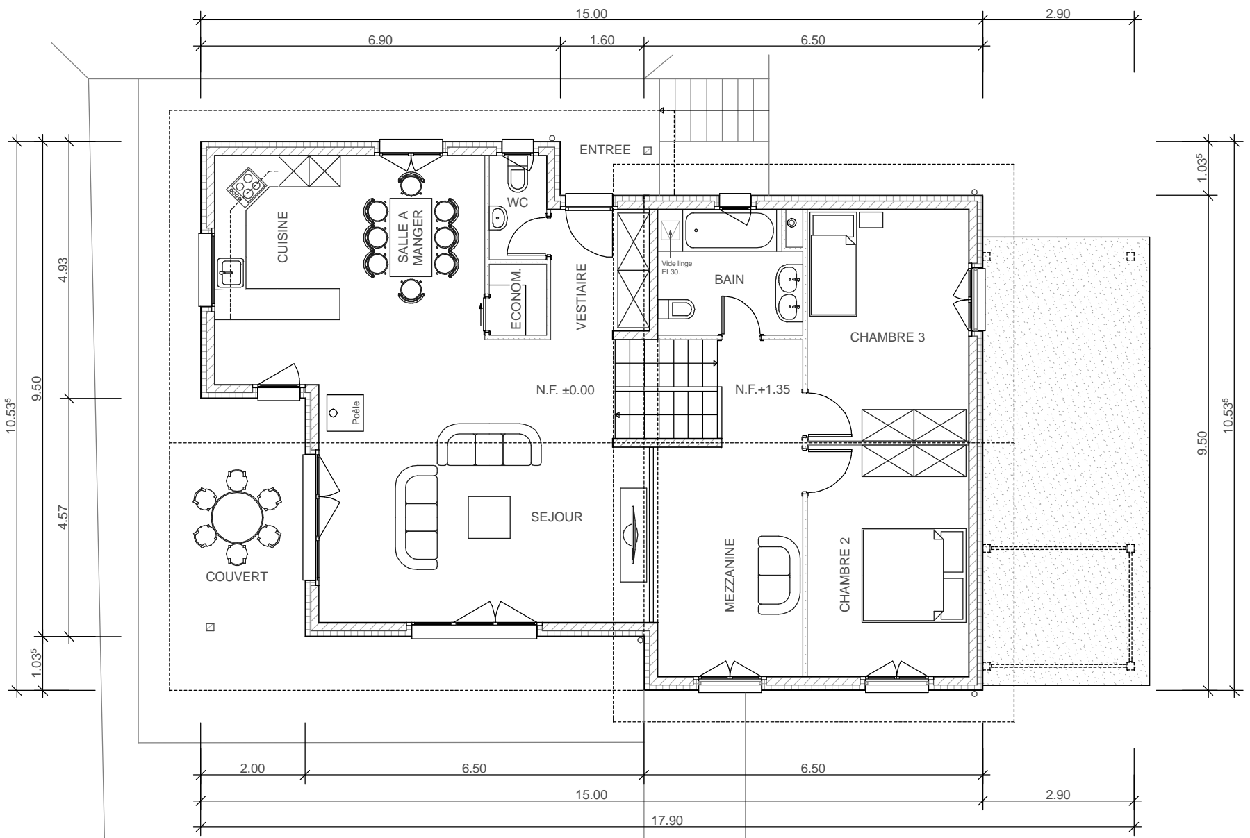
NIVEAUX DU REZ SUPÉRIEUR ET ÉTAGE 1:100
