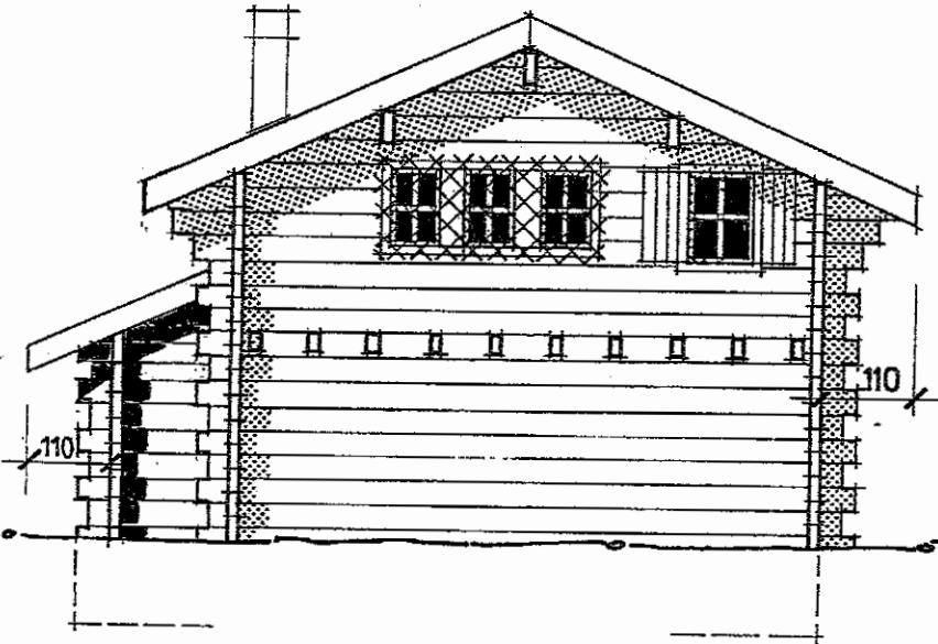
FACADE NORD
